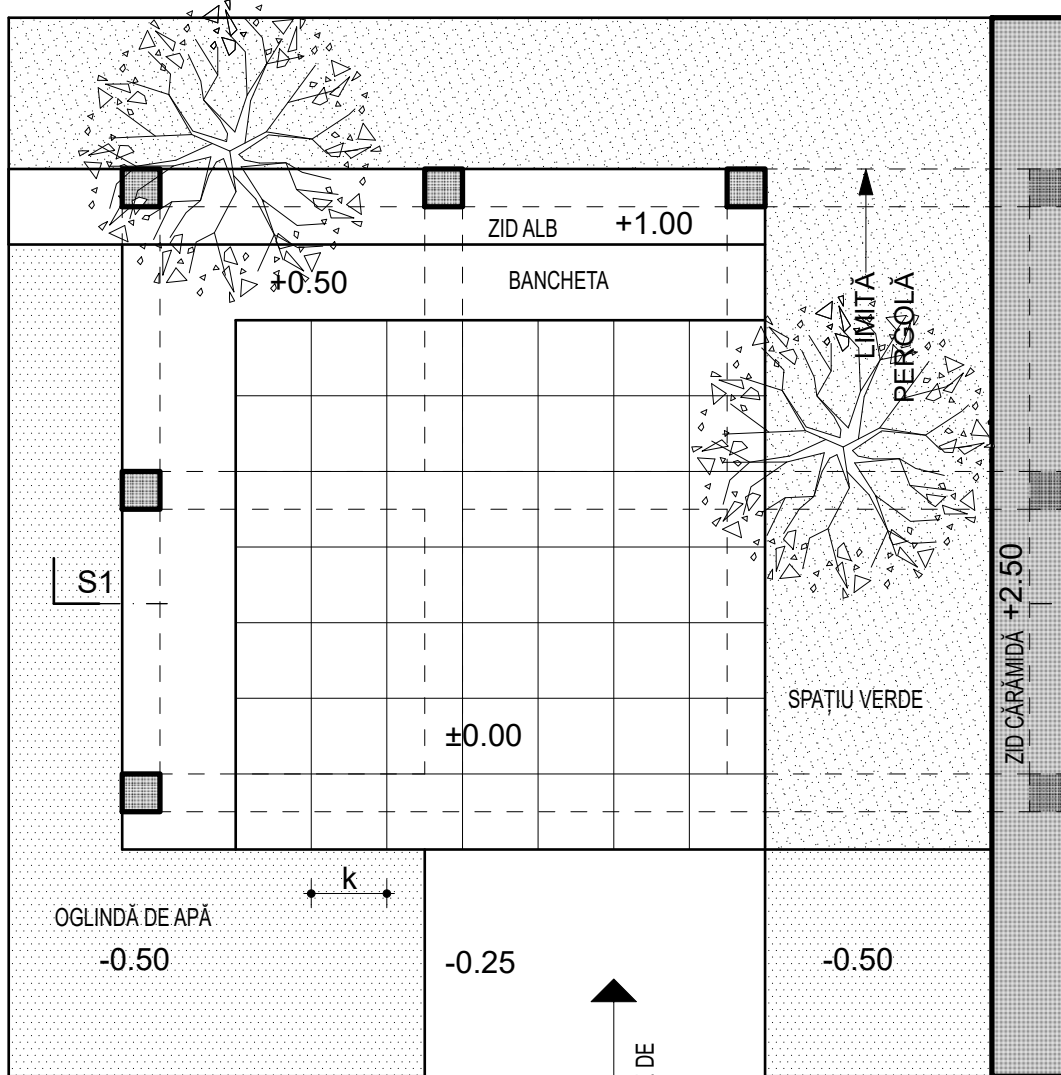
SECȚIUNE ORIZONTALĂ
