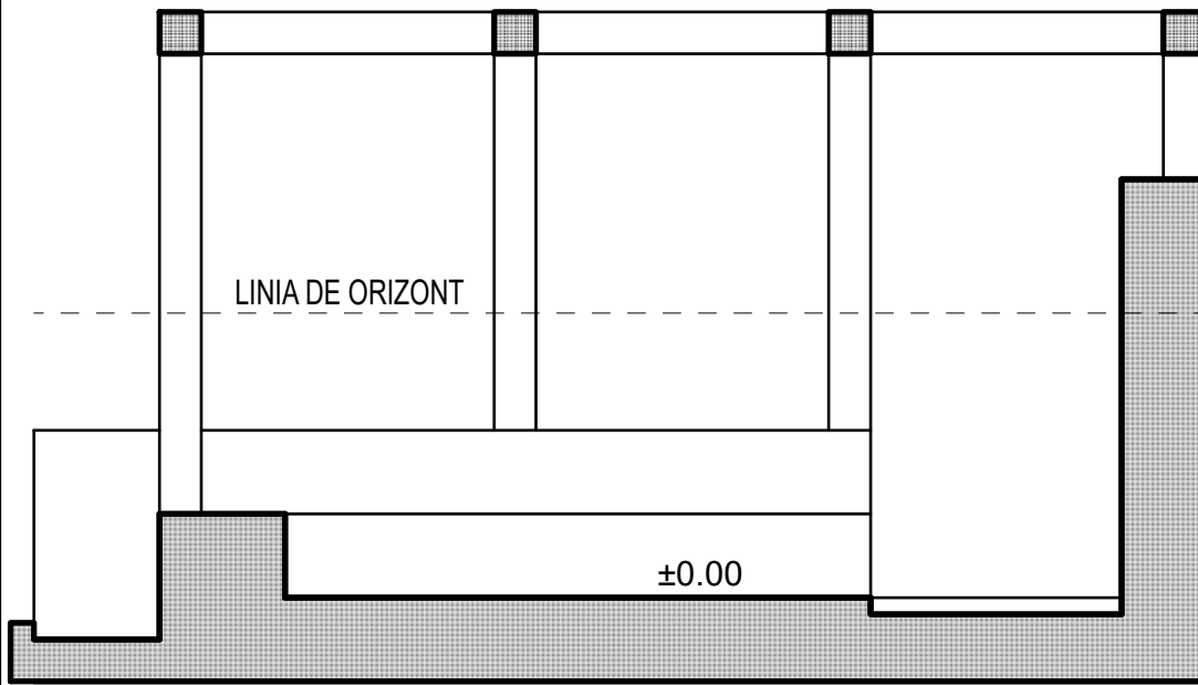
SECȚIUNE VERTICALĂ S1
